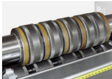
Ausführung für Steh- und Schnappfalz.
